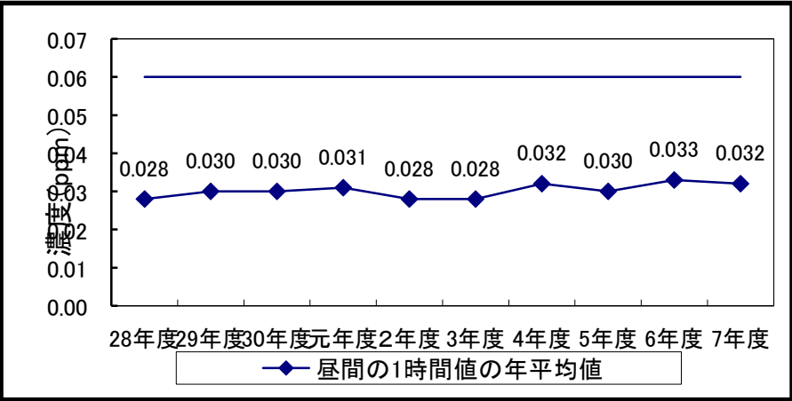
【図 5-5 川西市役所局光化学オキシダント濃度の経年変化（年平均値）】
