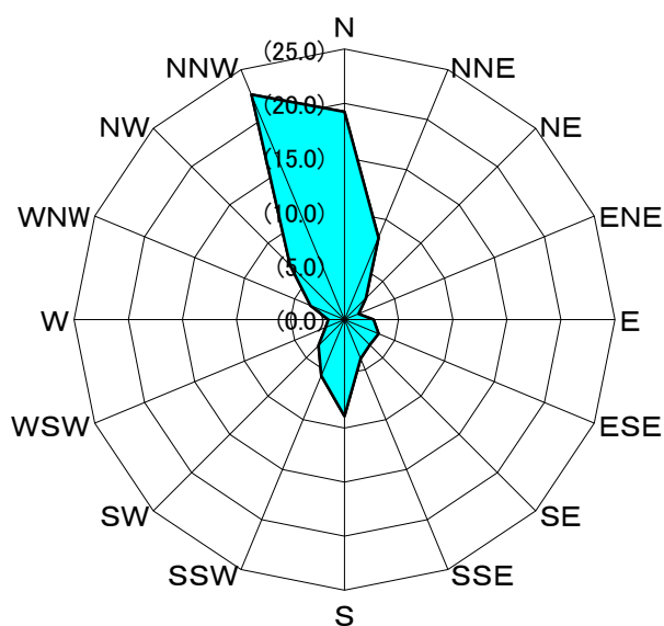
【図 5-7 令和7年度年間風配図 (川西市役所局)】
