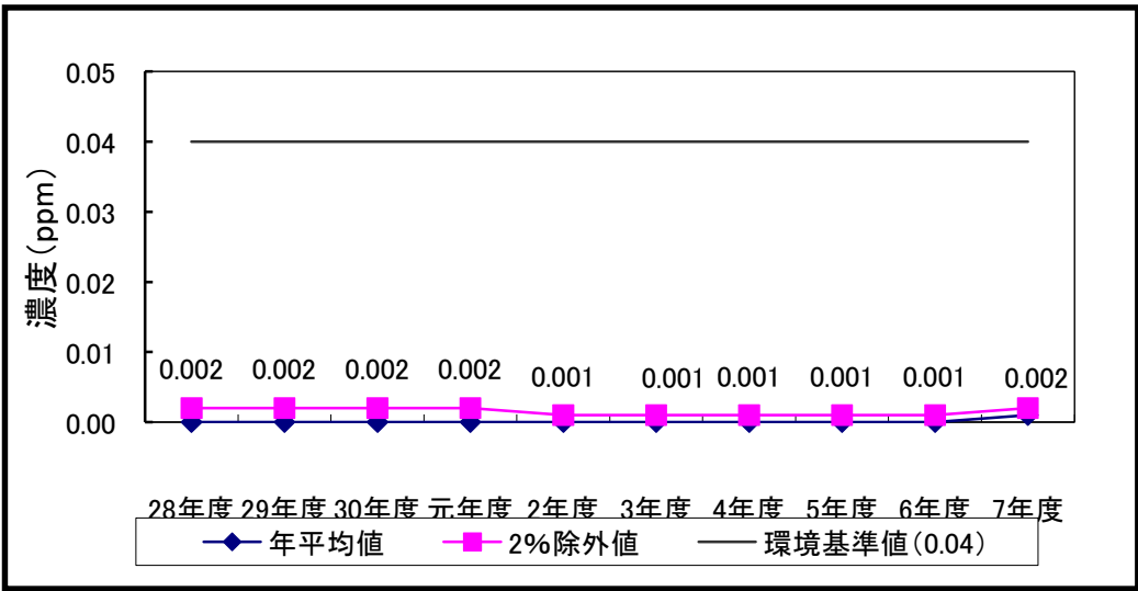
【図 5-2 川西市役所局二酸化硫黄濃度の経年変化（年平均値及び日平均値の年間2%除外値）】
