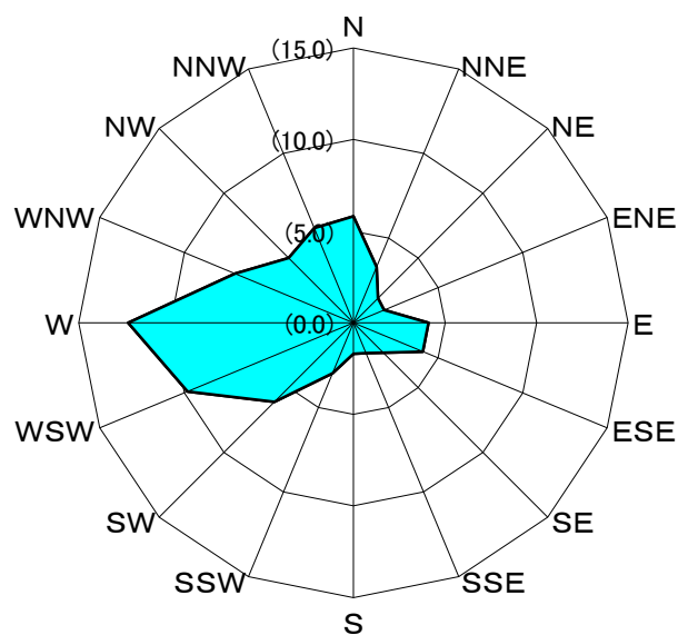
【図 5-15 令和7年度年間風配図 (川西文珠橋自動車排気ガス測定局)】
