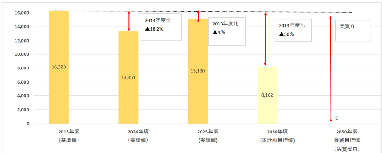
図1 温室効果ガス排出量の推移
