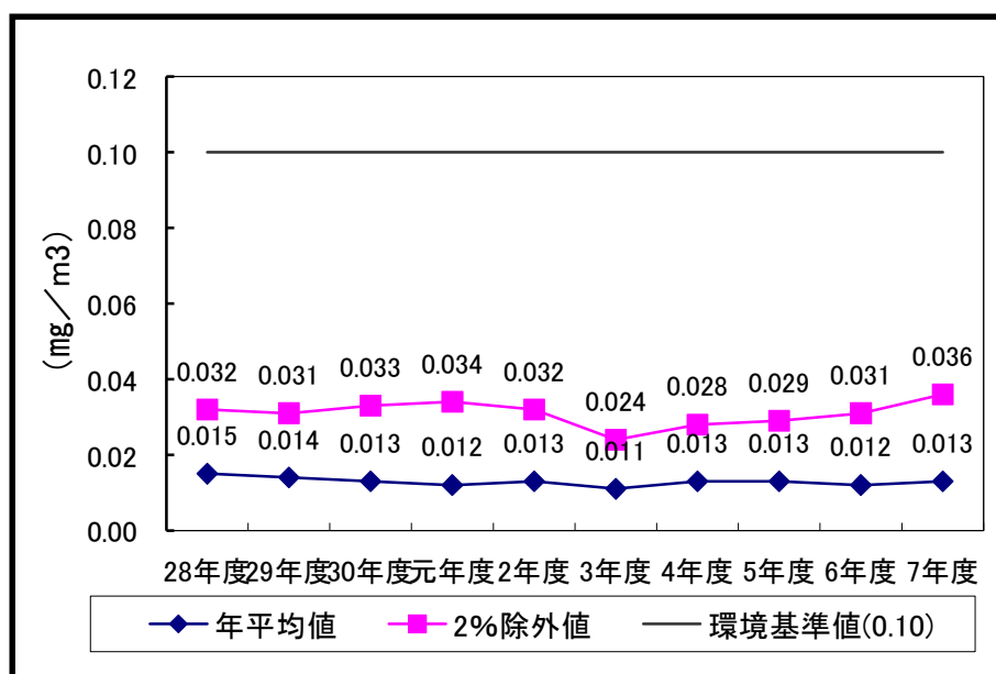
【図 5-3 川西市役所局浮遊粒子状物質濃度の経年変化 (年平均値及び日平均値の2%除外値)】
