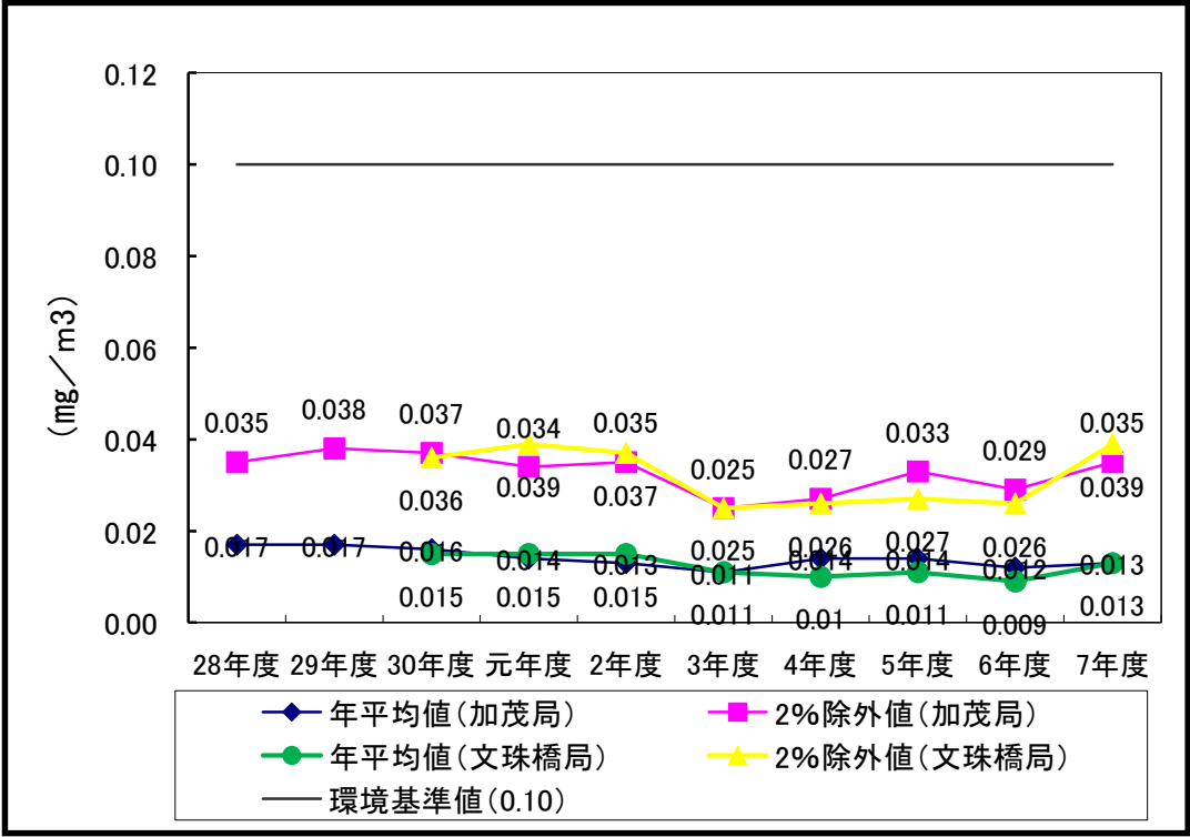
【図 5-11 加茂自動車排気ガス測定局と川西文珠橋自動車排気ガス測定局の浮遊粒子状物質濃度経年変化（年平均値及び日平均値の 2%除外値）】
