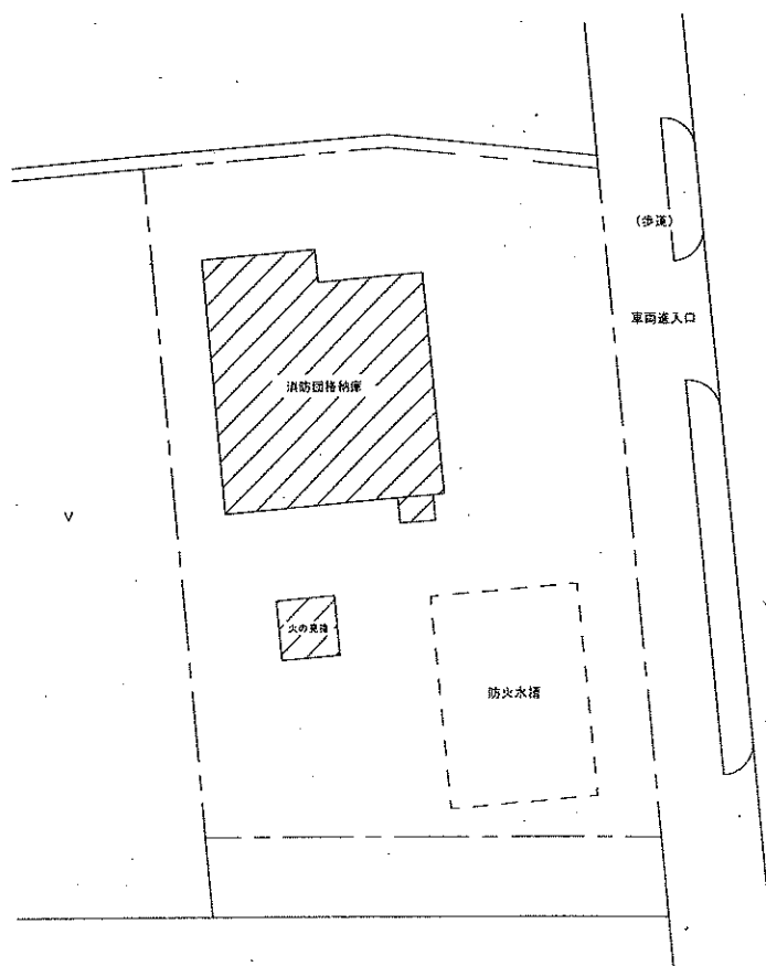
配置図 1/300
